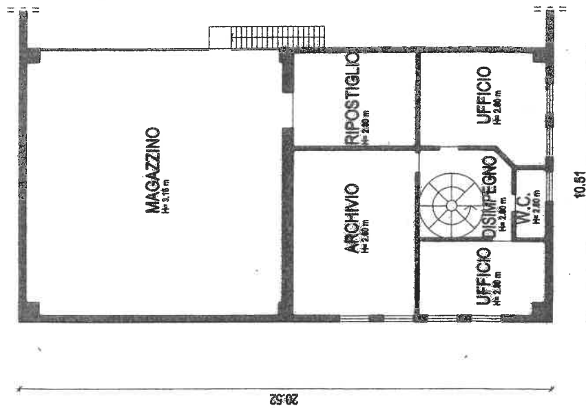
PIANO PRIMO H=2.80 - 3.15 m
