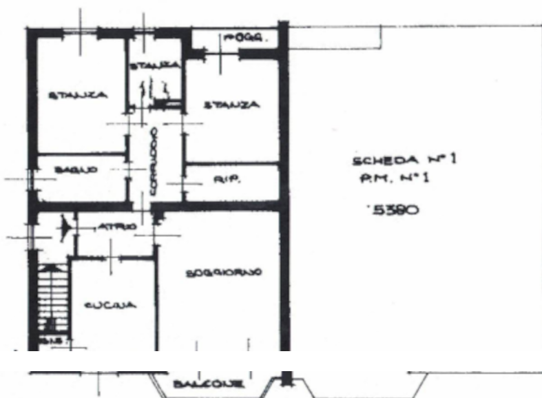
PIANTA PRIMO PIANO H = 2,70
