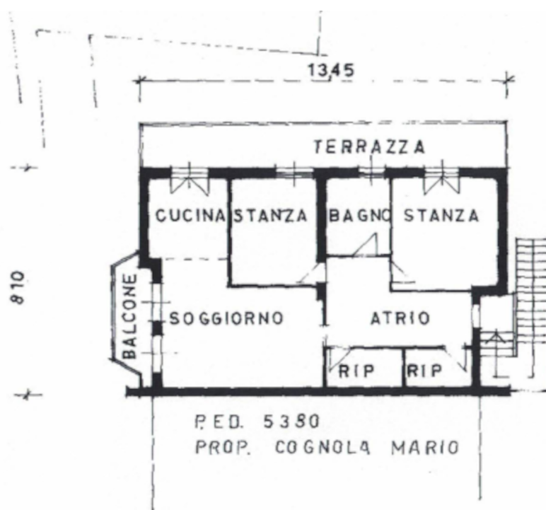
PIANTA 2° PIANO H= 810
